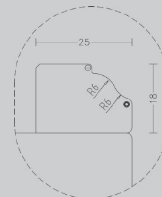
Legno interno in stile Barocco Internal wood in Baroque style
