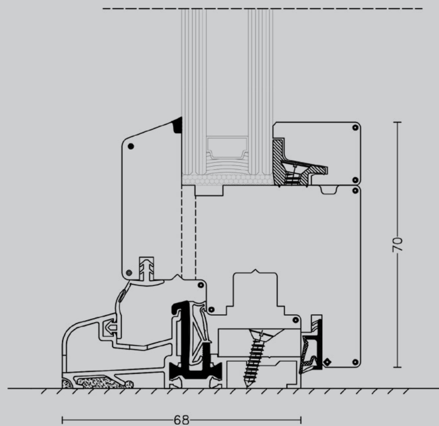
Portafinestra in legno con spessore anta 68x70 mm, interno in stile moderno, tripla guarnizione e doppio vetro. Wooden French window with shutter's thickness of 68x70 mm, in Modern style, triple seal and double glass.
