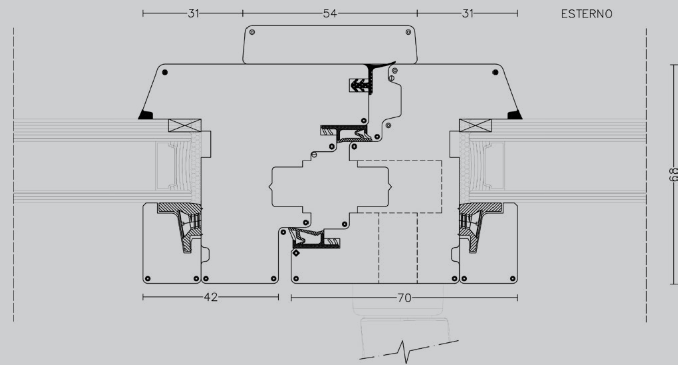
Finestra in legno con montante anta asimmetrico. Wooden window with asymmetric shutter's upright.
